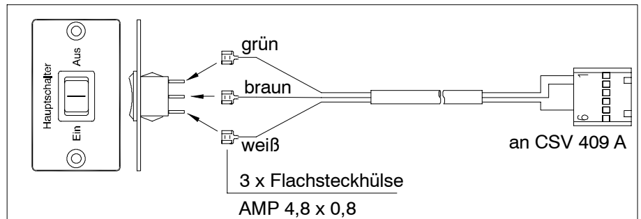
Bild 3 Anschluss Verbindungskabel an ST 05
