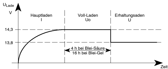
Bild 6 Beispiel für den Ladespannungsverlauf mit dem Caravan-Ladesystem CSV 409 A
