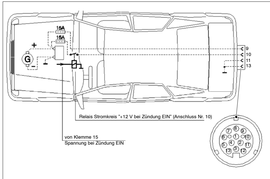
Bild 4 Anschluss Steckdose Zugfahrzeug
