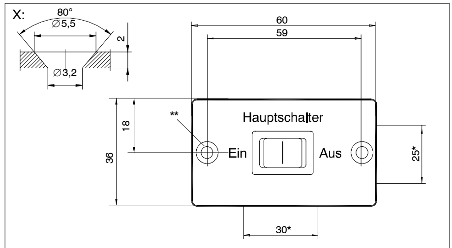
Bild 2 Maßbild Schalttafel ST 05 (Abmessungen in mm) * Möbelausschnitt, Einbautiefe inklusive Flachsteckhülsen ca. 30 mm ** 2 x Senkung, siehe Einzelheit X
