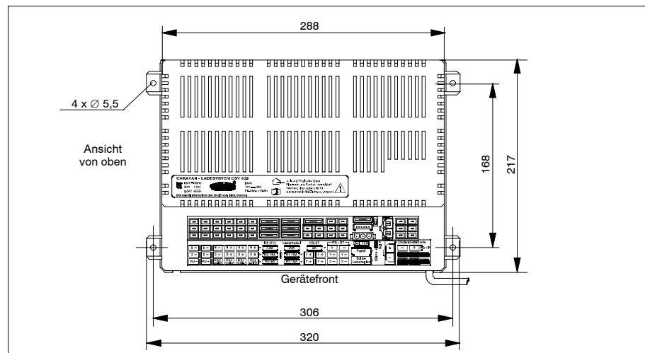
Bild 1 Maßbild Caravan-Ladesystem CSV 409 A (Abmessungen in mm)
